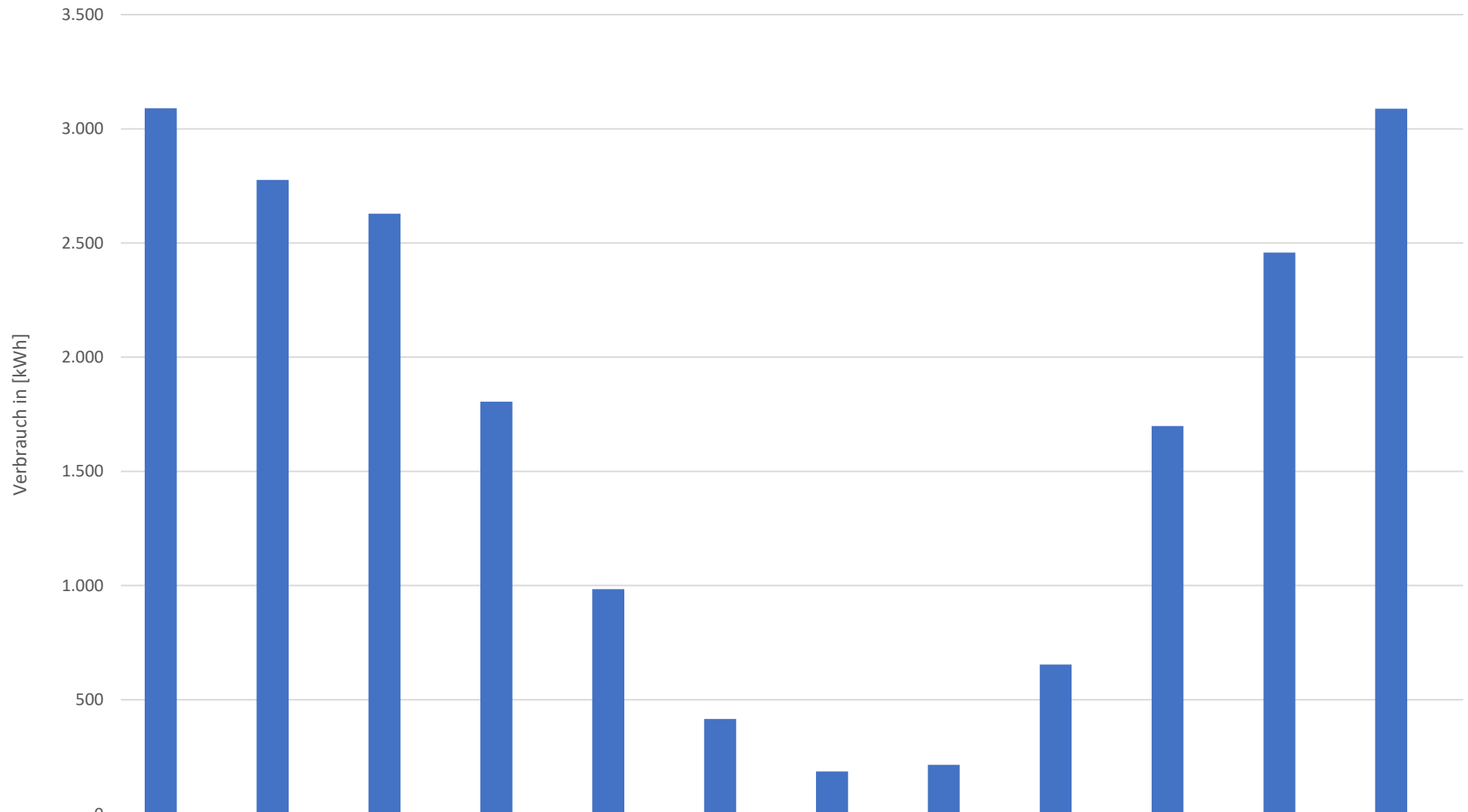
Jährliche Verteilung des Erdgasverbrauchs eines Einfamilienhauses (20.000 kWh pro Jahr)
